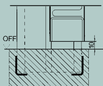
Замыкание двери без упора, серийно
