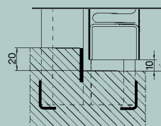
Замыкание двери с упором, под заказ или обеспечивается заказчиком на месте
